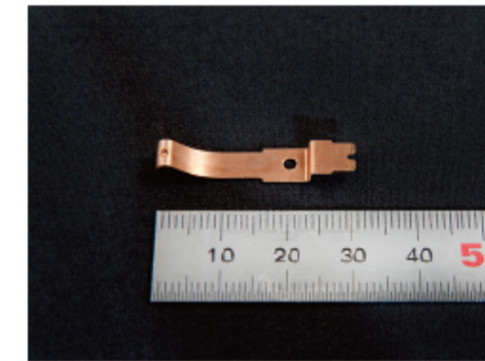
ターミナル [りん青銅 T=0.5mm]
