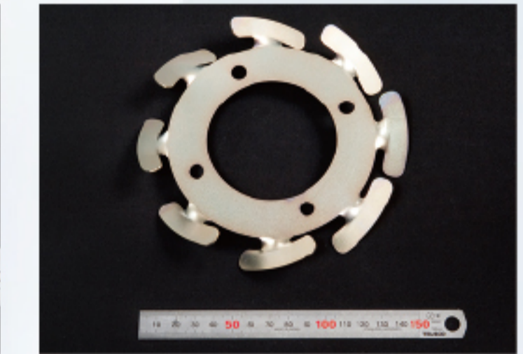
ファン [SPCC T=1.2mm]
