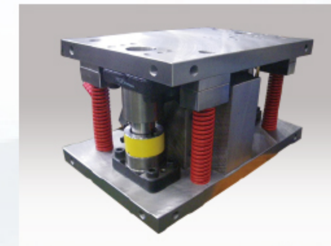
単型 [斜め切断型]
