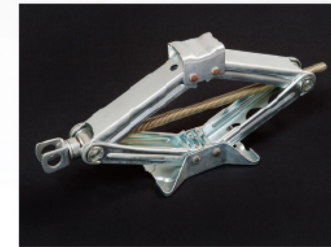
自動車用ジャッキ試作品 [SPHC T=1.6~2.6mm]
