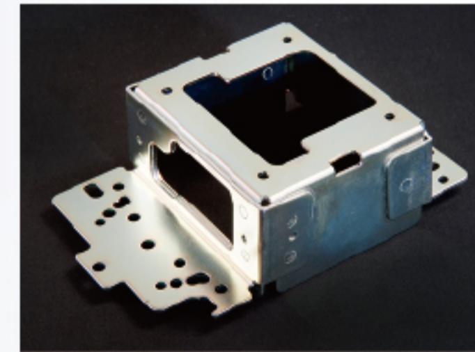
ブラケット [SPCC T=1.2mm]
